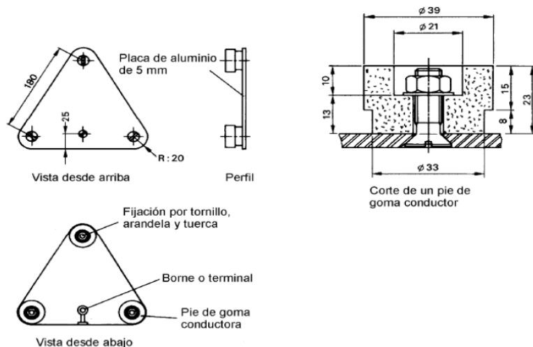
Figura 19.1.1 – Electrodo de ensayo 1
