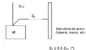
Figura 2. Conductores de equipotencialidad entre una masa M y una estructura
