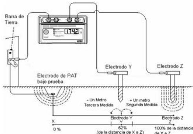
Figura 1. Método de la caída de potencial para medir la RPT
