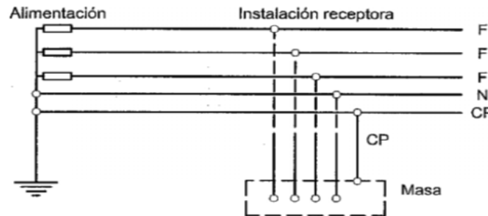
Figura 5.1 Esquema TN-S
