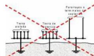
Figura 3. Puesta a tierra separadas o independientes
