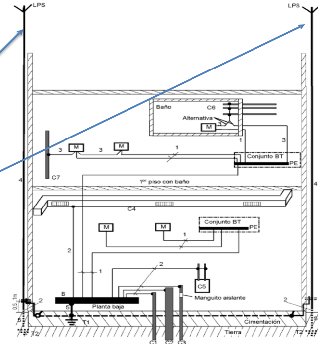
ILUSTRACIÓN DE UNA DISPOSICIÓN DE PUESTA A TIERRA, CONDUCTORES DE PROTECCIÓN Y CONDUCTORES DE EQUIPOTENCIALIDAD
