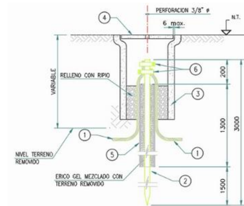
DETALLE CONEXION BARRA COPPERWELD EN CAMARA DE REGISTRO
