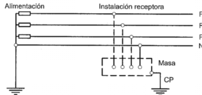
Figura 5.4 Esquema TT
