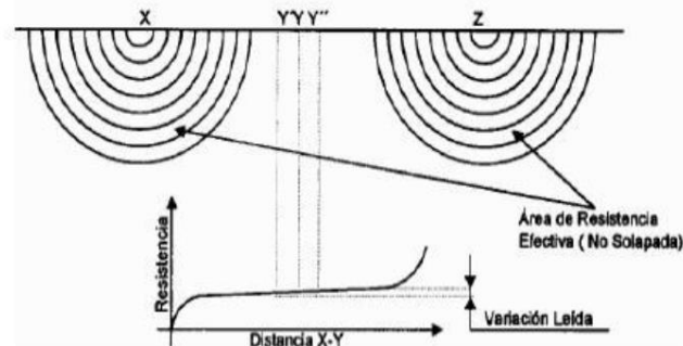
Figura 4. Curva de resistencia versus distancia sin superposición de gradientes de potencial
