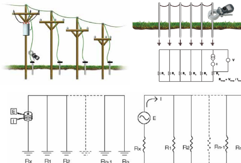
Figura 6. Circuito equivalente para un sistema puesto a tierra en más de un punto
