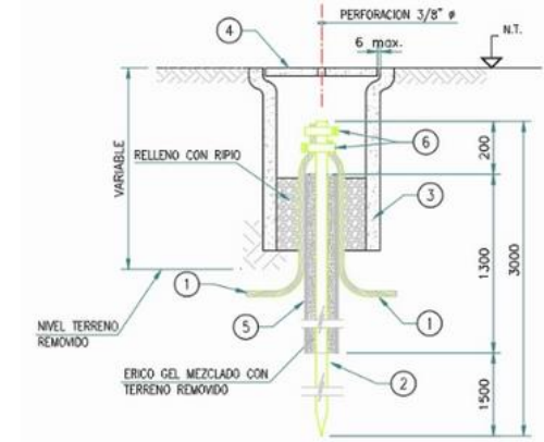
DETALLE CONEXION BARRA COPPERWELD EN CAMARA DE REGISTRO
