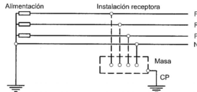
Figura 5.4 Esquema TT
