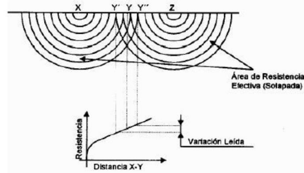
Figura 3. Superposición de los gradientes de potencial
