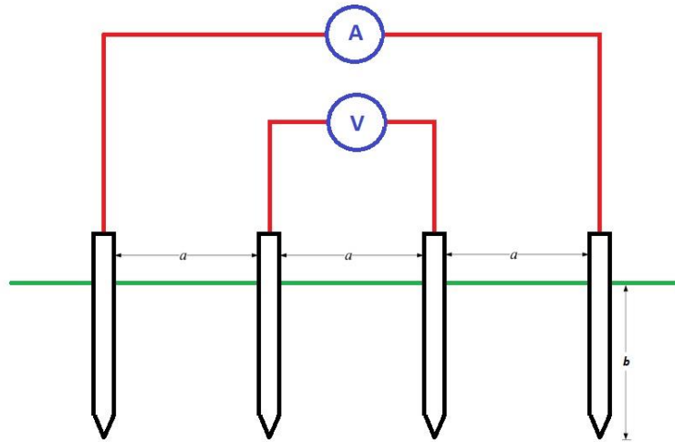
WENNER
