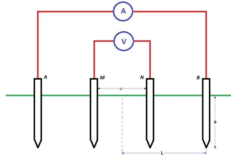
SCHLUMBERGER
