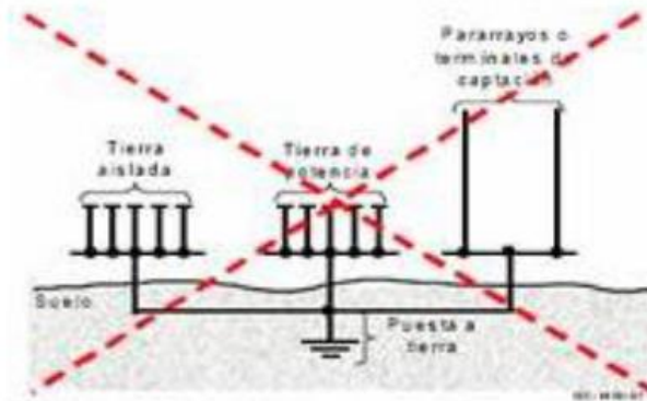
Figura 2. Una sola puesta a tierra para todas las necesidades
