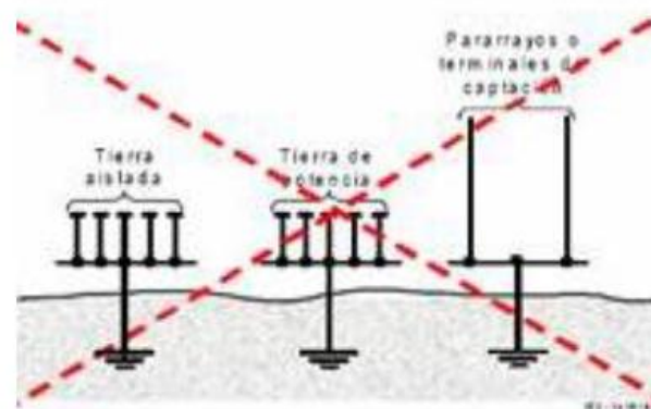
Figura 3. Puesta a tierra separadas o independientes
