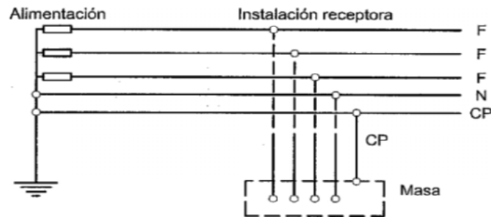
Figura 5.1 Esquema TN-S
